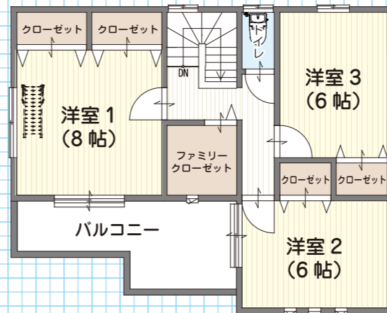
2階平面図
